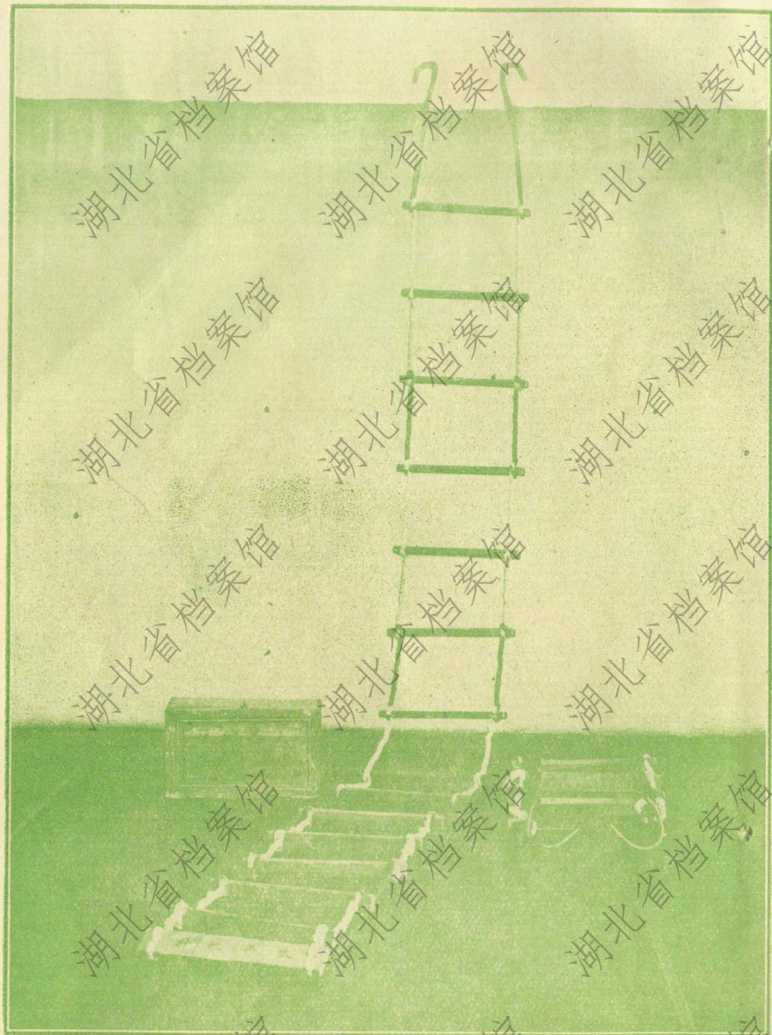
太平梯軟梯掛圖(1) 太平梯軟梯捲藏圖(2) 太平梯軟梯裝入錦盒圖(3)
