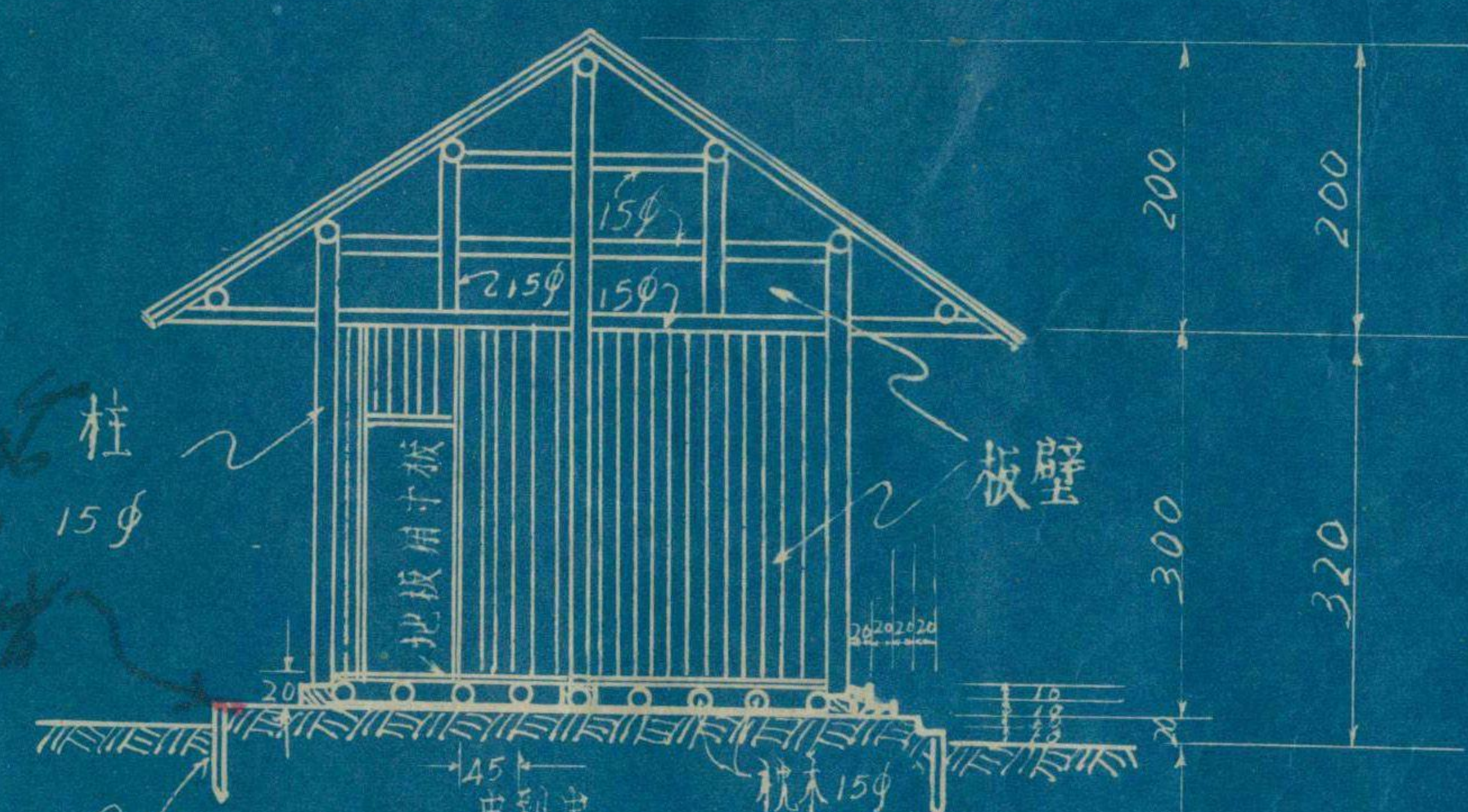
甲甲剖面圖
