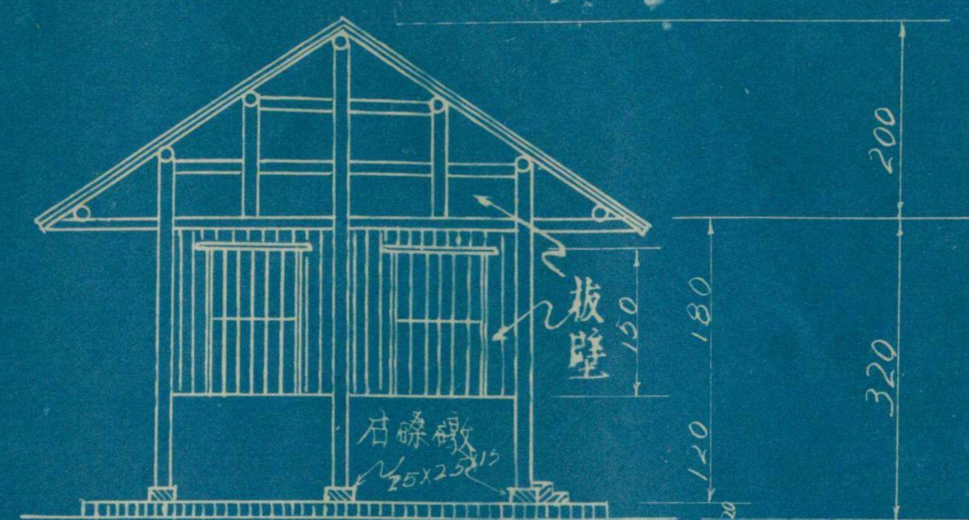
側面圖
