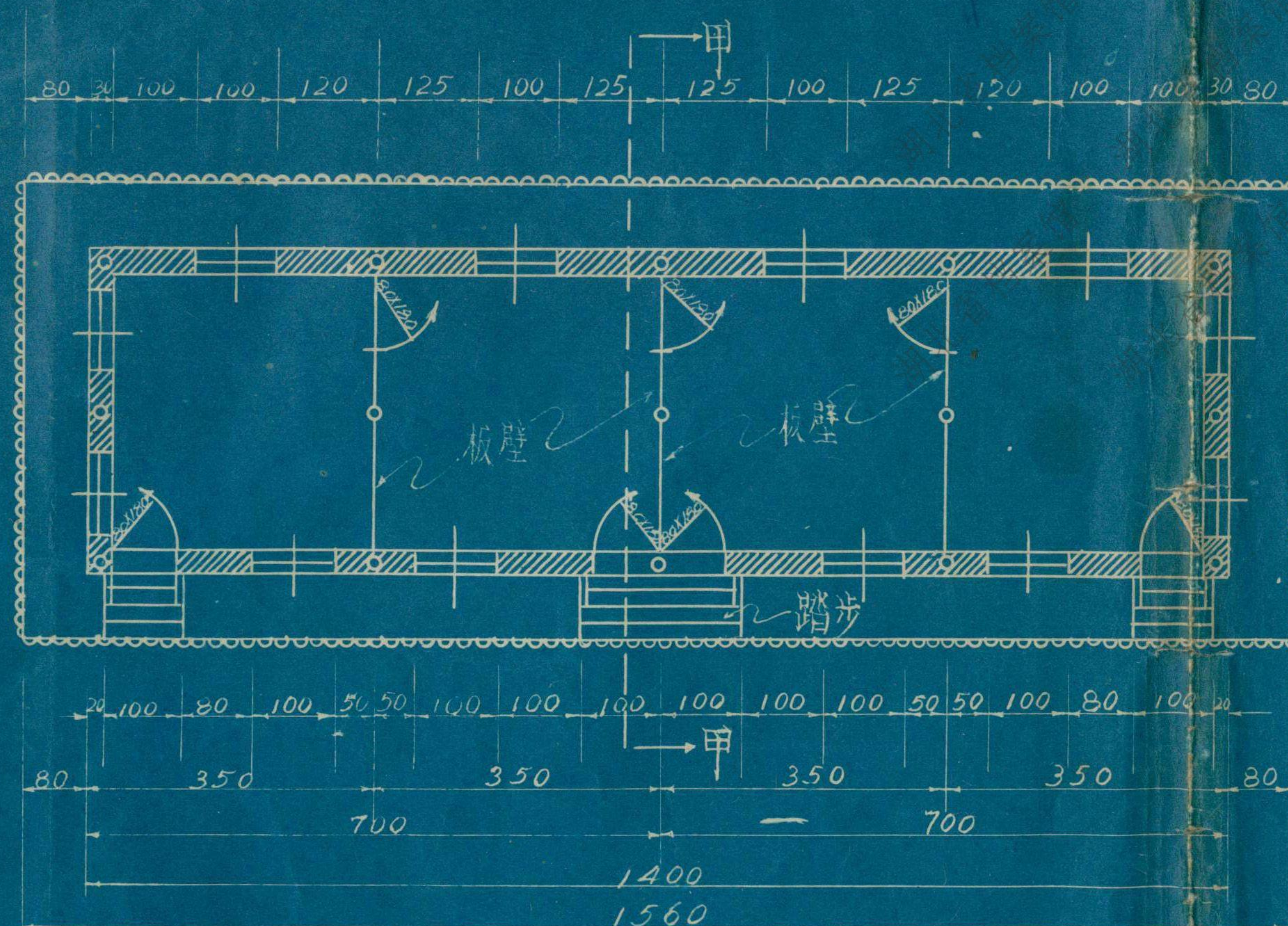
平面圖
