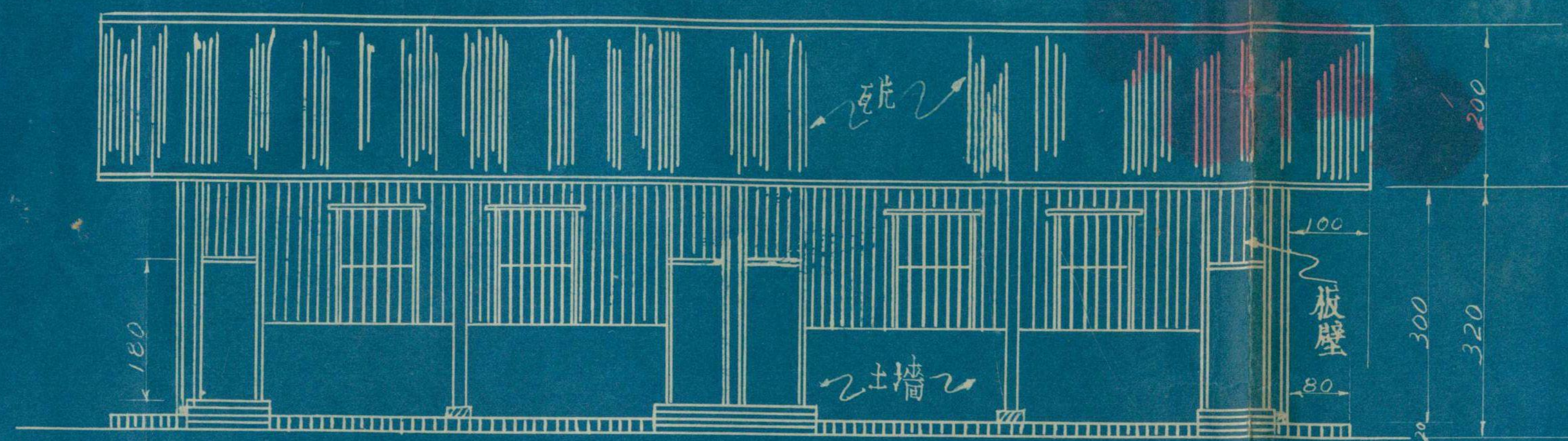
正面圖
